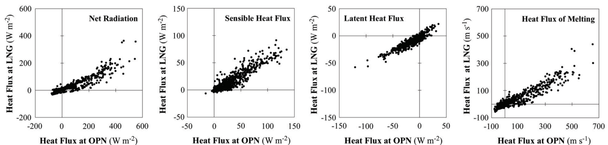
図1 開地(OPN)と林内(LNG)における正味放射量、顕熱フラックス、潜熱フラックス、融雪熱量の関係
