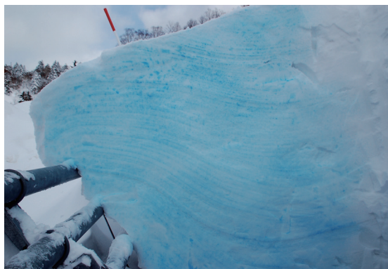
写真7 雪庇の断面構造
