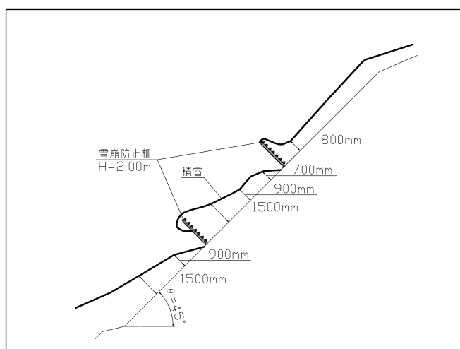
図 1 斜面積雪分布
